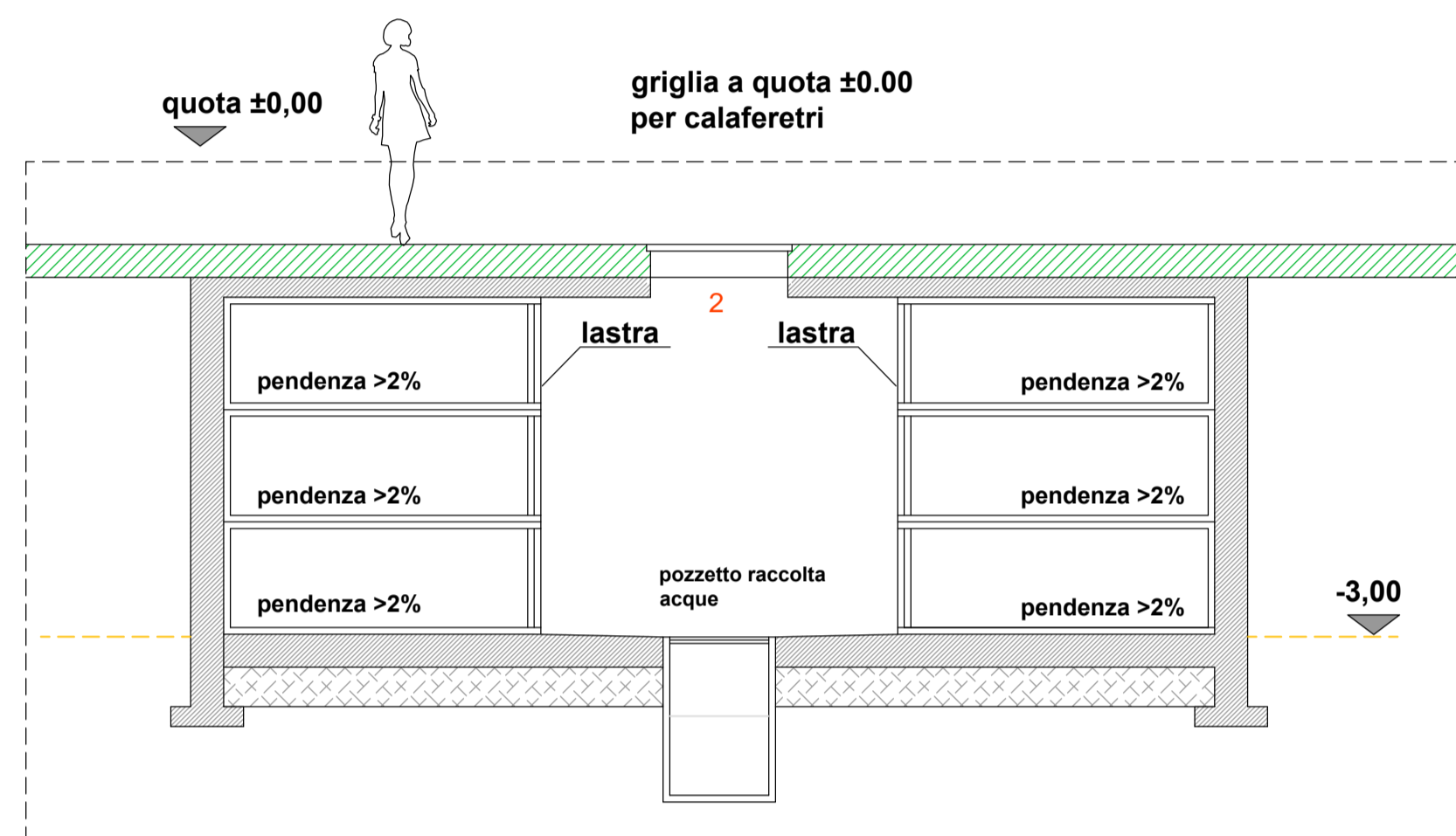
Tomba famiglia interrata vestibolo centrale Sezione tipo
